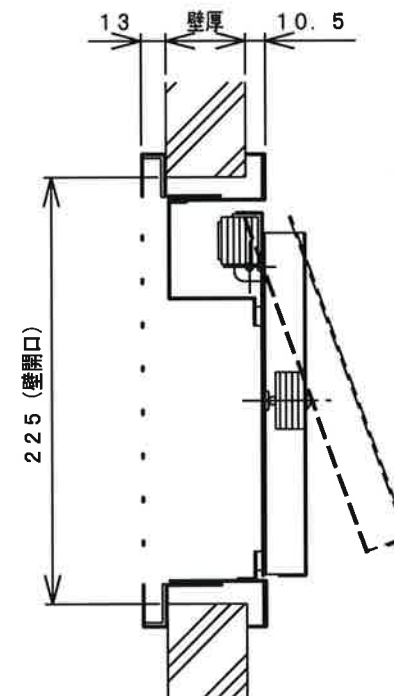
A-A断面
