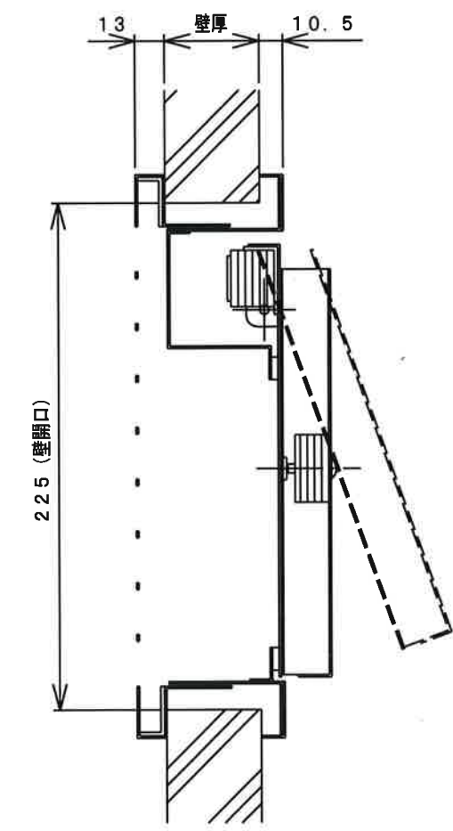
A-A断面
